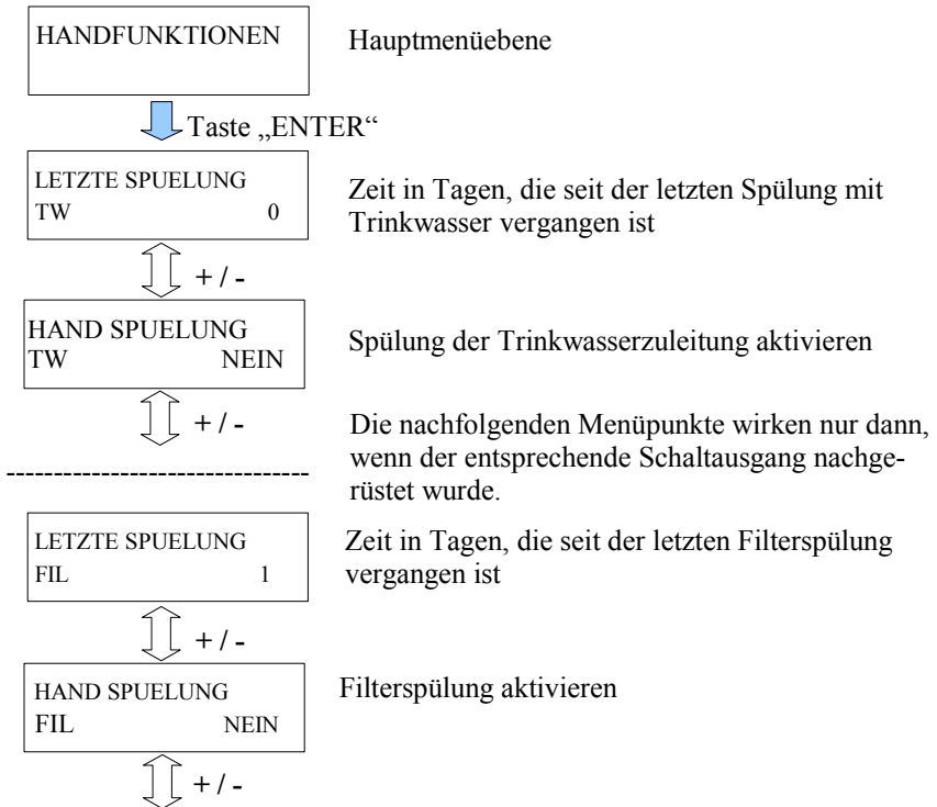
Abbildung 12: Untermenü „Handfunktionen“
