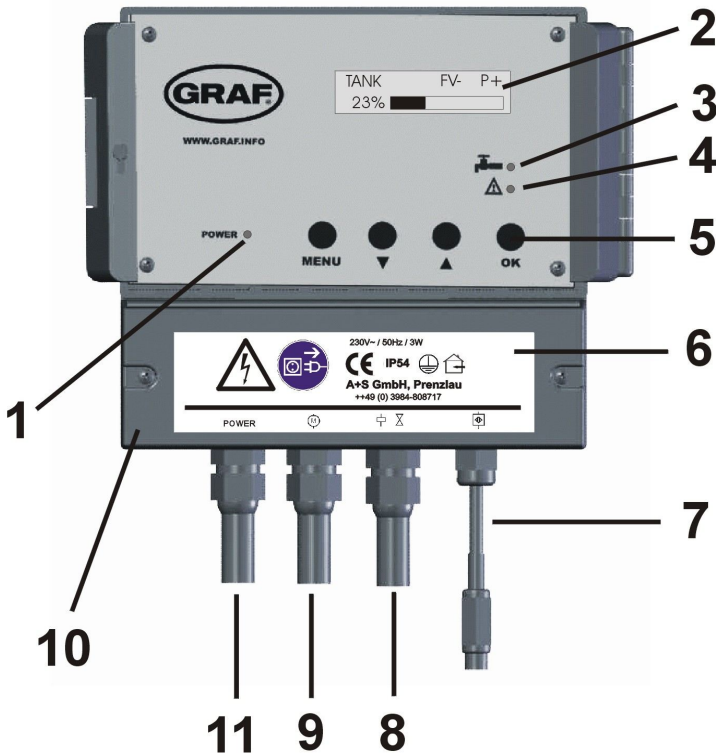
Abbildung 1: Geräteansicht
