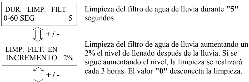
Figura 10: Submenú "Puntos de conmutación"
