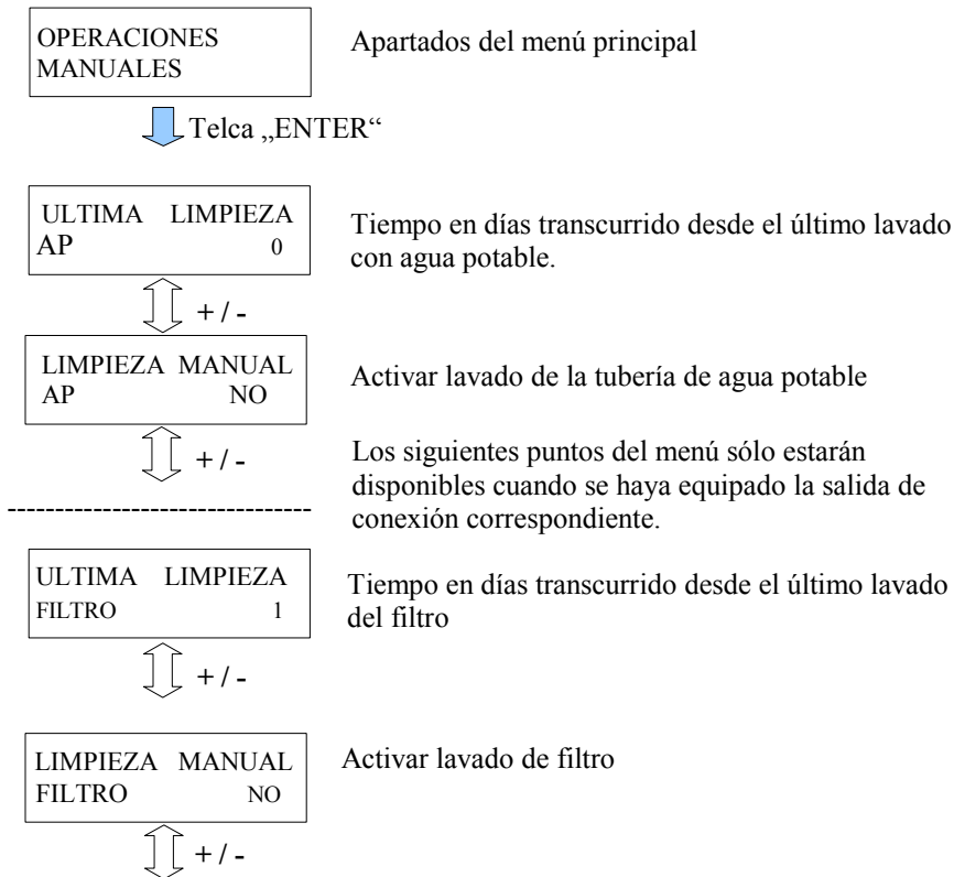
Figura 12: Submenú "Funciones manuales"
