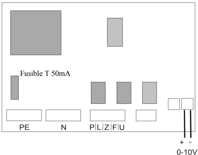
Ilustración 19: Ubicación de la salida analógica
