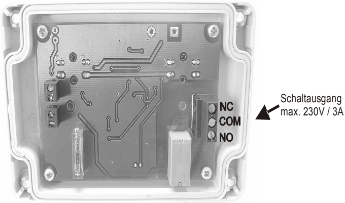
Abbildung 5: Schaltausgang
